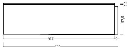
COLONNE COLUMNS
